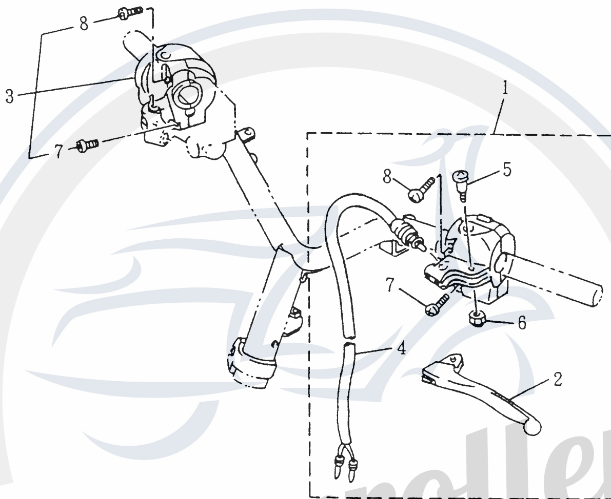
Modelle mit Scheibenbremse
