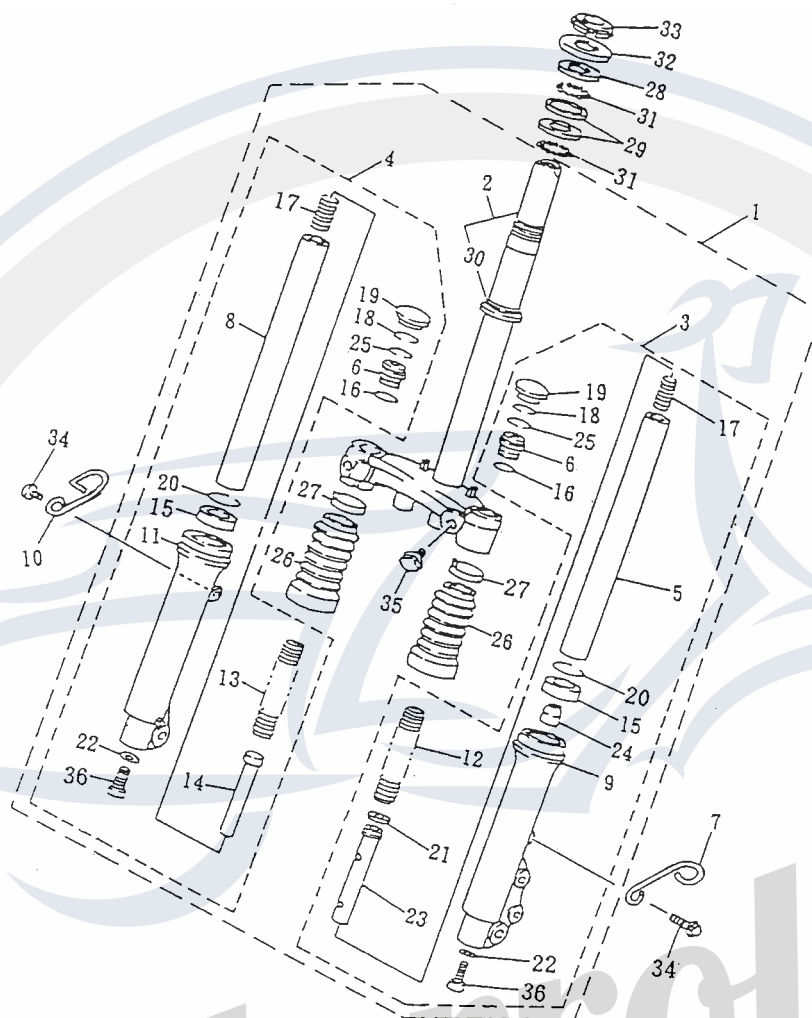
Modelle mit Scheibenbremse
