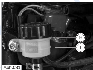
Bremsflüssigkeitsbehälter Hinterradbremse
