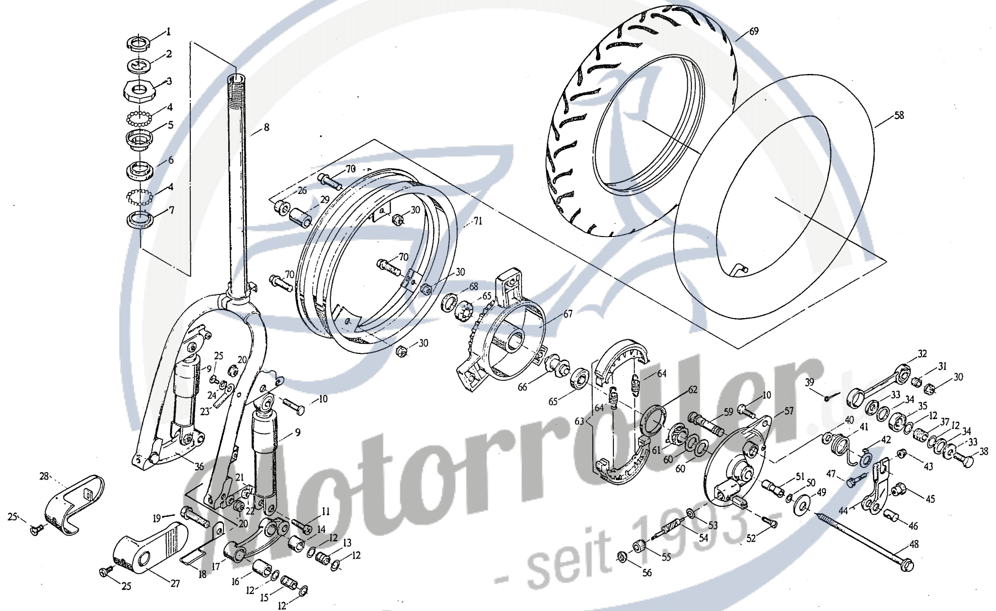
Fig. 8 Vorderrad-Federung Vorderrad
