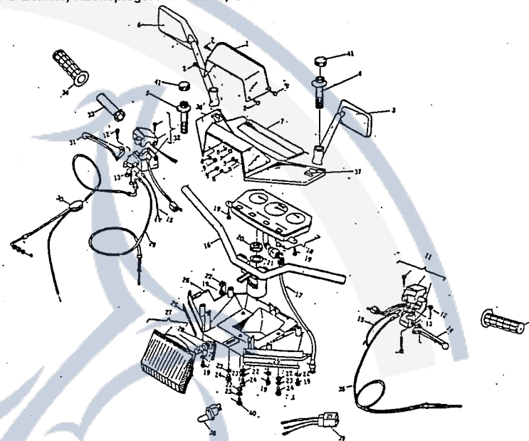
Fig. 9 Lenker, Rückspiegel Armaturen, Scheinwerfer
