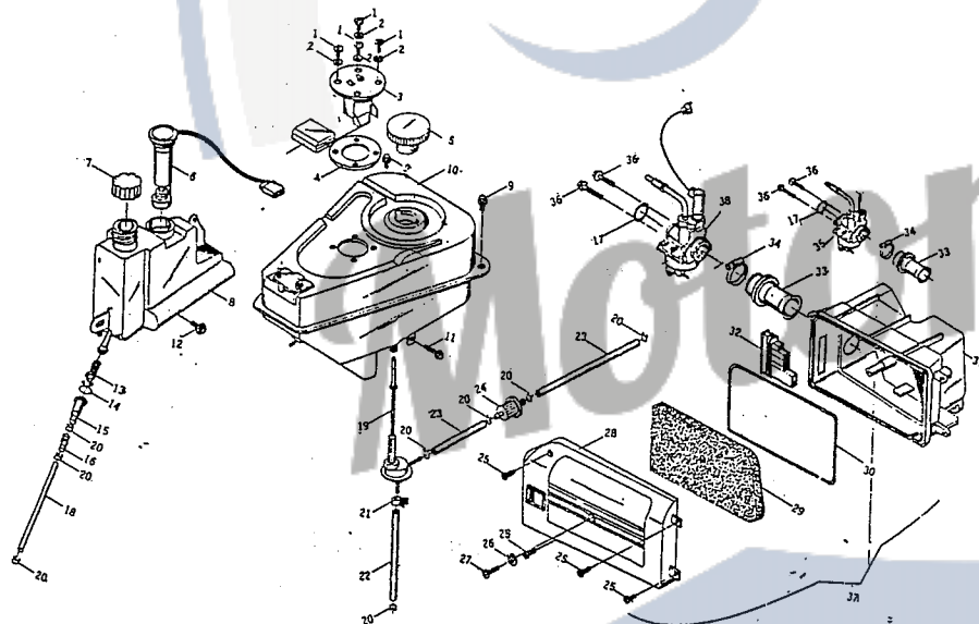
Fig. 5 Kraftstofftank Benzinhahn Öltank Vergaser Luftfilter
