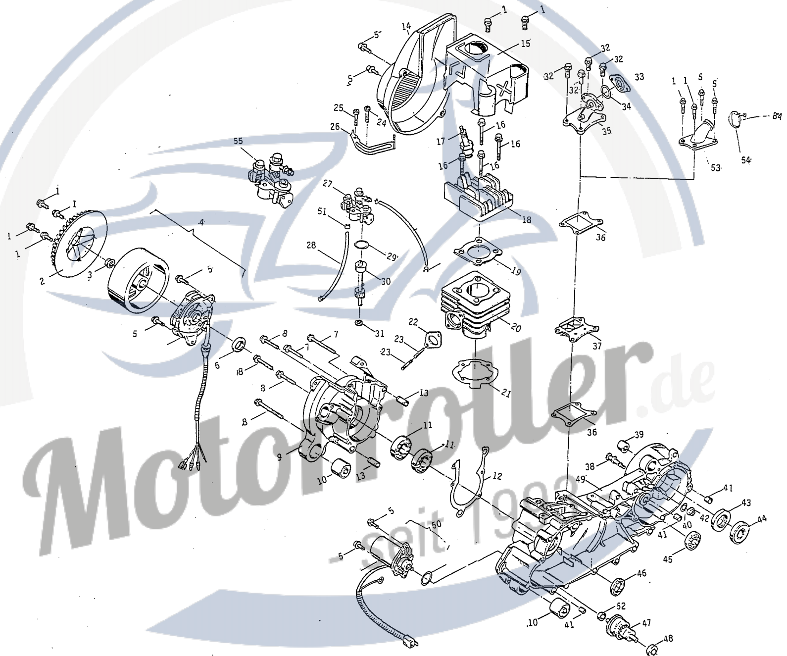
Fig. 1 Kühlgebläse Zylinder Zylinderkopf Lichtmaschine Kurbelgehäuse Ölpumpe
