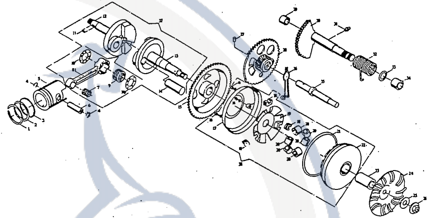
Fig. 3 Kolben Kurbelwelle Vorderer Variomatik
