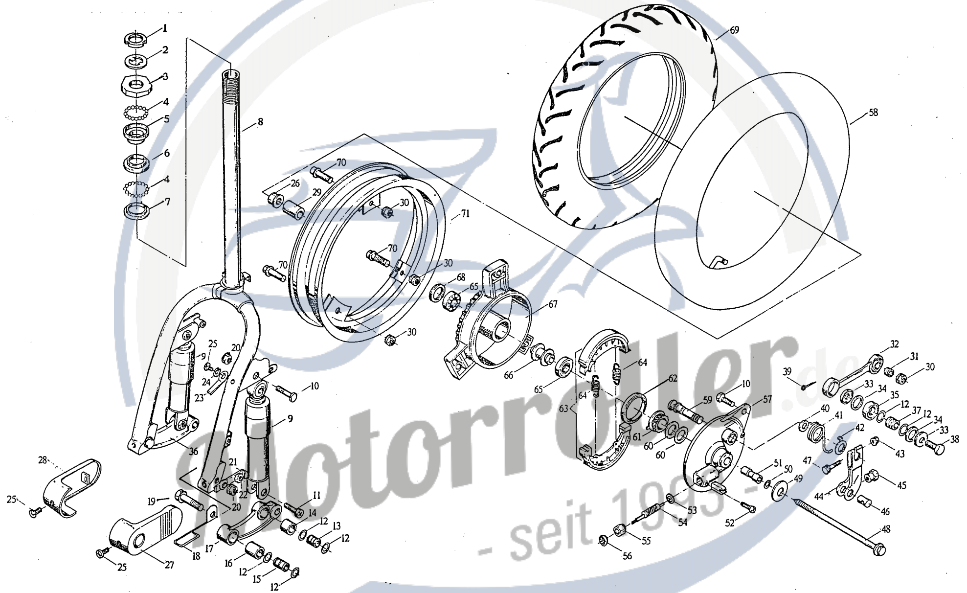
Fig. 8 Vorderrad-Federung Vorderrad
