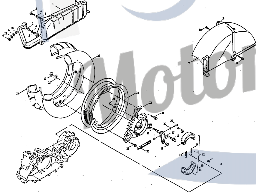
Fig. 2 Auspuff Hinterrad
