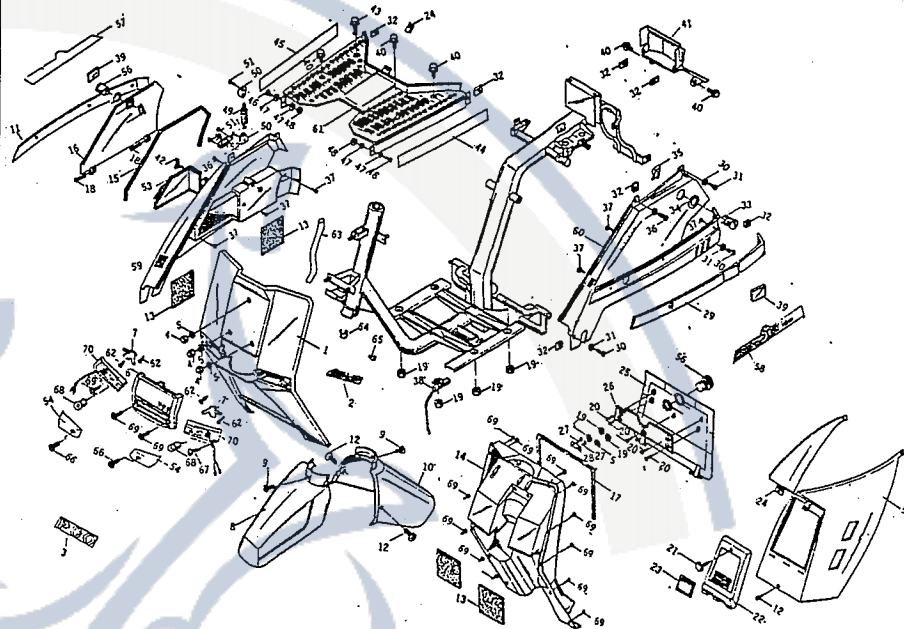
Fig. 6 Verkleidungsteile
