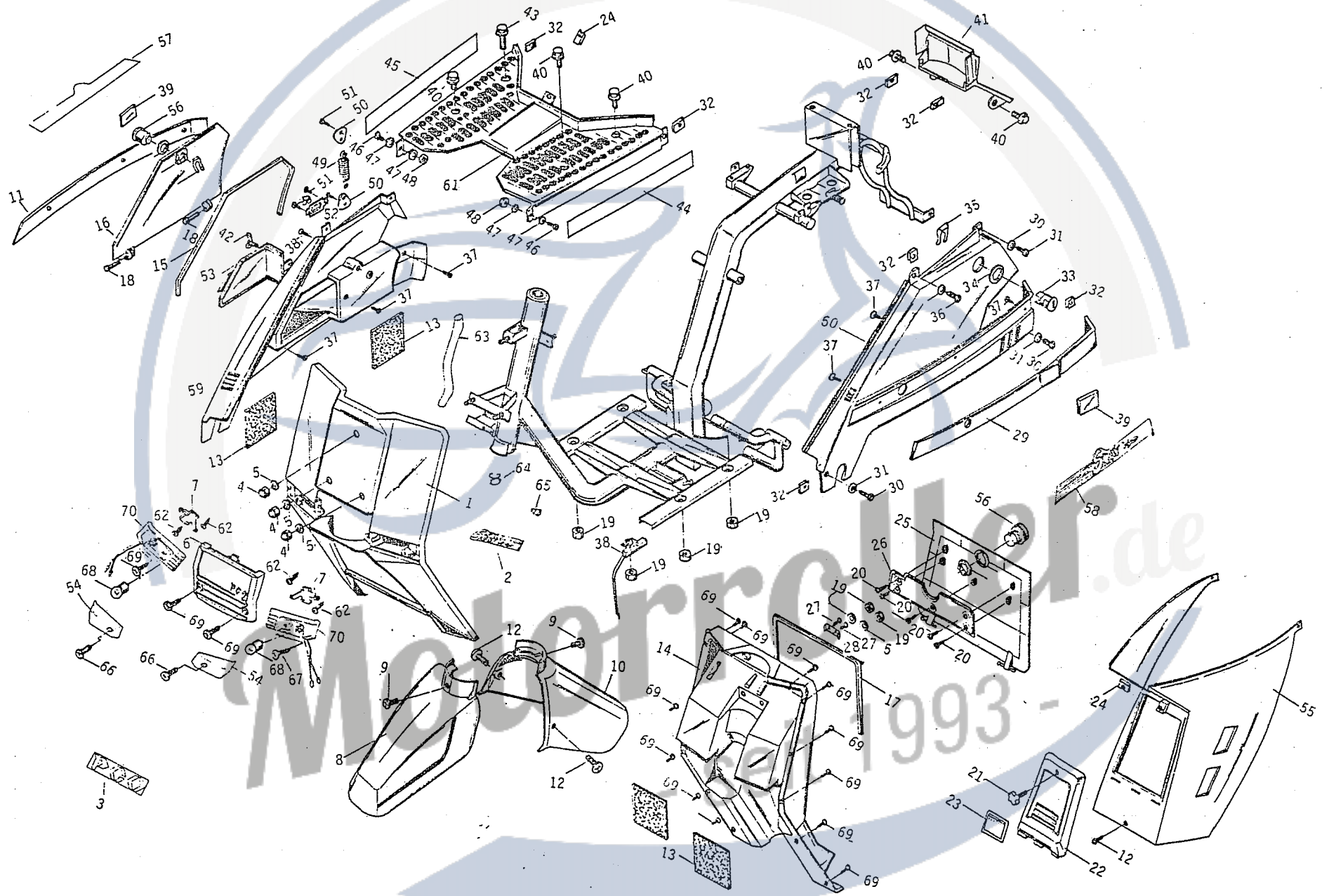
Fig. 6 Verkleidungsteile
