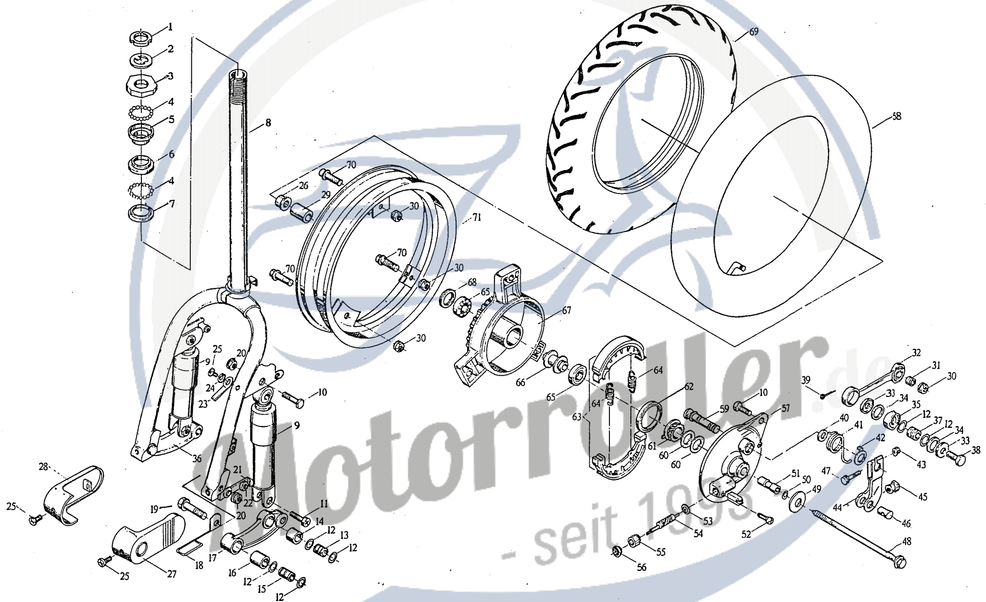
Fig. 8 Vorderrad-Federung Vorderrad
