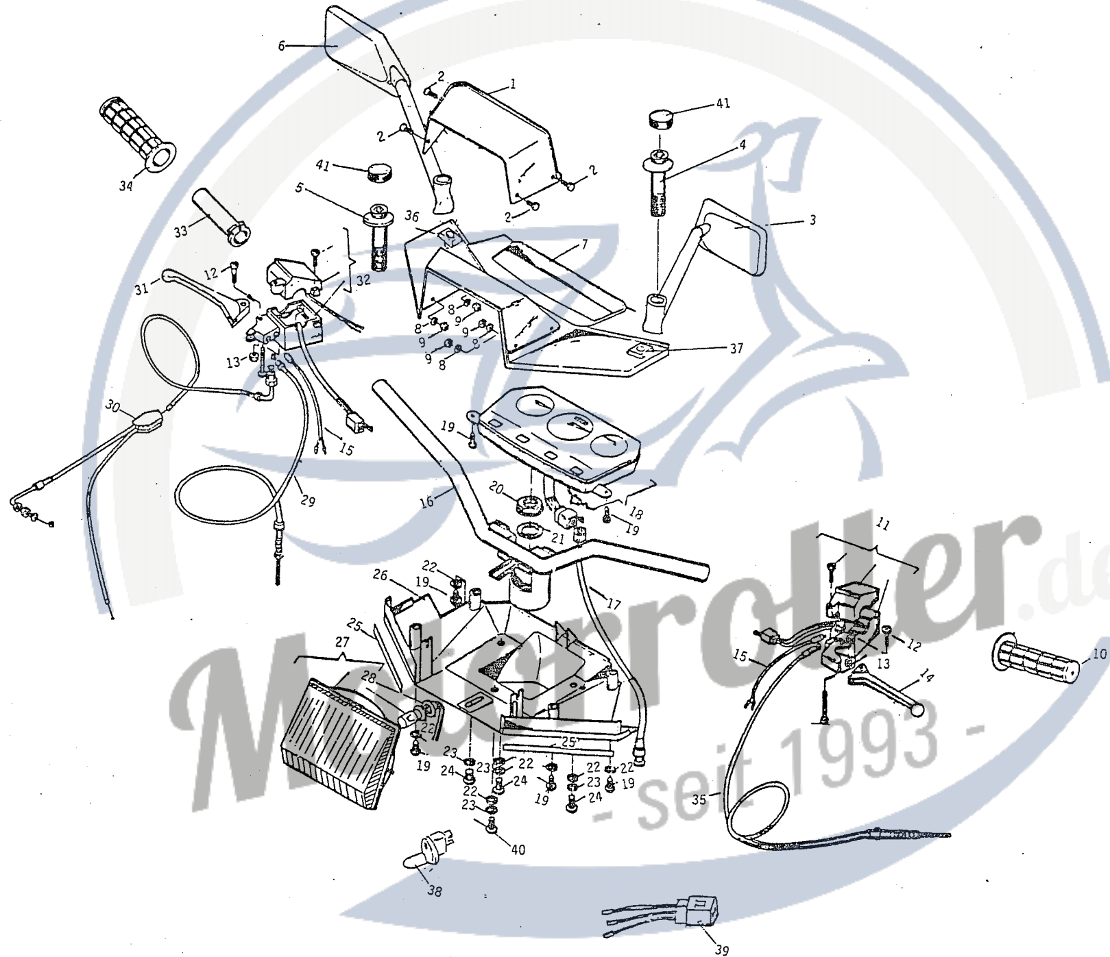
Fig. 9 Lenker, Rückspiegel Armaturen, Scheinwerfer
