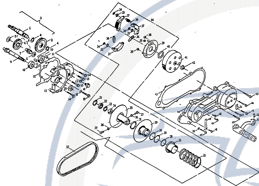
Fig. 4 Variomatik Seitendeckel Kickstarter Hinterradgetriebe
