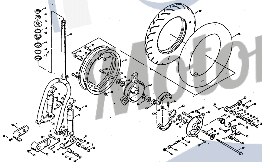
Fig. 8 Vorderrad-Federung Vorderrad
