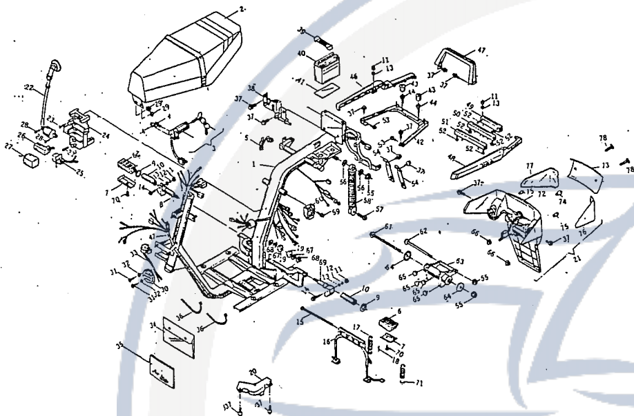
Fig. 7 Elektr Ausrüstung Sitz Gepäckträger Ständer Rahmen
